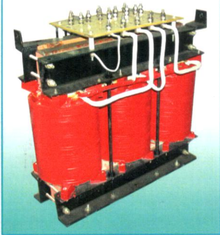
20 KVA Resin Cast
