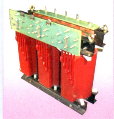
100 KVA Resin Cast
