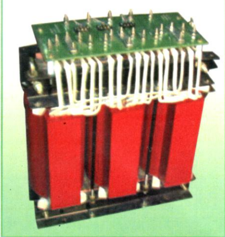
20 KVA Resin Cast
